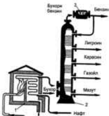
Расми 20. Оташдони луладор ва манораи ректификатсионӣ
