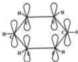
Нақши ҳосилшавии \pi -бандҳо аз p -абрҳои электронӣ
