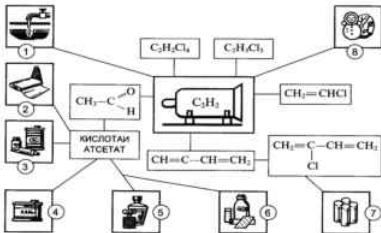
Расми 15. Истифодабарии атсетилени ва пайвастҳои он: 1-барои кафшер ва буридани металҳо; 2-ҳосил кардани нахи сунъӣ; 3-рангубор; 4-лакҳо; 5-атр ва моддаҳои атторӣ; 6-дорувор; 7-каучуи хлорпренӣ; 8-поливинилхлорид.
