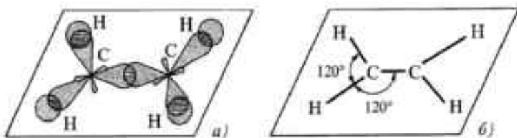
Расми 8. Нақшаи ба вучуд омадани σ-бандҳо дар молекулаи этилен.
