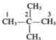
n-пентан (ҳарорати ҷӯшиш 36,2^\circ C )
