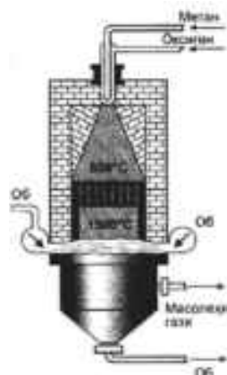
Расми 14. Ҳосил кардани атсетилени аз метан
