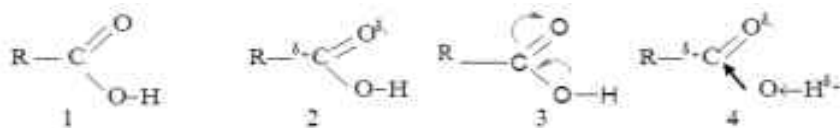
Формулаи кислотаҳои яқини сари карбонӣ.
