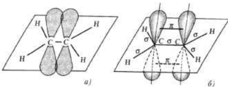
Расми 9. Схематик пайдоиши \pi -банд дар молекулаи этилен
