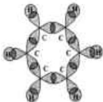
Нақши ҳосилшавии \sigma -бандҳо ( C-C ва C-H )
