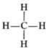
формулаи структурии метан
