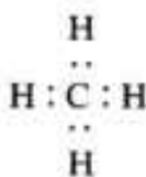
формулаи электронии метан
