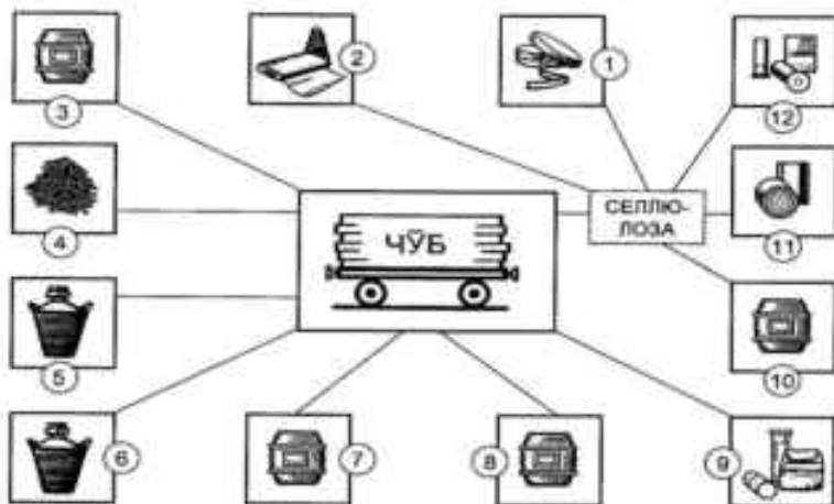
Расми 32. Маҳсулотҳои коркарди химиявии ҷӯб: 1 – ҳосил кардани кинонаворҳо; 2 – нахҳои сунӣ; 3 – скипидар; 4 – ангишти ҷӯб; 5 – кислотаи сирко (атсетат); 6 – спирти метил; 7 – канифол; 8 – зифт; 9 – глюкоза; 10 – хӯроки чорво; 11 – қоғаз; 12 – борутӣ бедуд.
