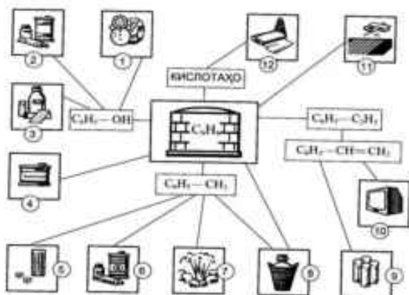
Расми 19. Истифодаи бензол, ҳомологҳои он ва пайвастҳои онҳо: 1,10-ҳосил кардани массаҳои пластикӣ; 2,6-рангуборҳо; 3- доруворӣ; 4-анилин; 5-сахарин; 7-моддаҳои тарканда; 8-ҳалқунан- даҳо; 9-каучуи бутадиенстиролӣ; 11-пестицидҳо; 12-нахи лавсан.
