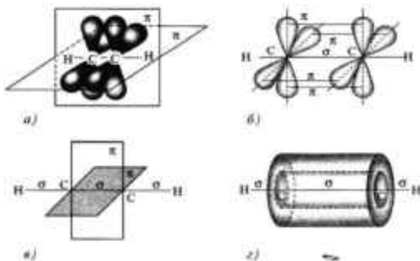
Расми 13. Нақшаи ба вуҷуд омадани \pi -банд дар молекулаи атсетилен: а, б-ҷуфт-ҷуфт пушида шудани абрҳои p -электронҳо; в-ду сатҳи ба ҳам перпендикуляр, ки дар он \pi -бандҳо ба вуҷуд меоянд; г-абри силиндрӣ \pi -электронҳо дар атсетилен.
