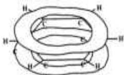
\sigma -ва \pi -бандҳо дар молекула
