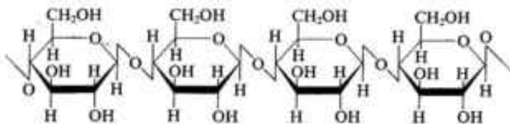
Порча (фиқра)-и молекулаи селлюлоза
