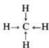
майли чуфти умумии электронҳо
