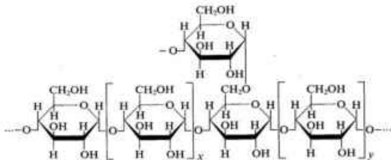
Порча (фиқра)-и молекули крахмал
