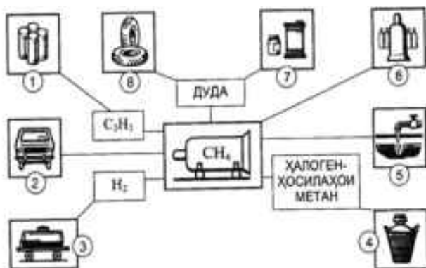
Расми 7. Истифодаи метан ва маҳсулотҳои он: 1-ҳосил кардани каучуи синтезӣ; 2-сӯзишворӣ барои муҳаррикҳои дарунсӯз; 3-ҳосил кардани бензини синтезӣ; 4-истеҳсоли ғалқунандаҳо; 5-барои буридан ва васл кардани металлҳо; (филизот) 6-ба сифати сӯзишворӣ; 7-истеҳсоли ранг барои матбаа; 8-истеҳсоли резин.
